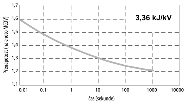
INZIP trenutna prenapetostna krivulja
