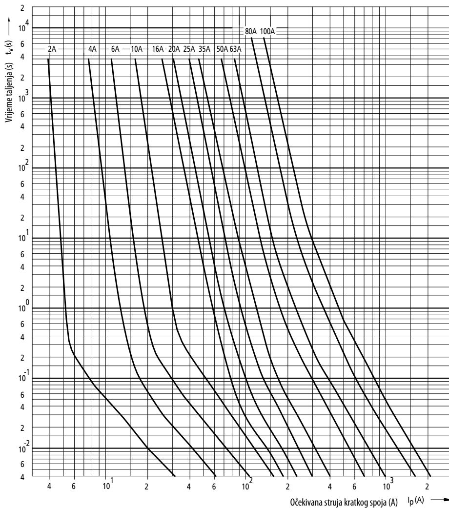
Vremensko-strujna karakteristika I/t DZ
