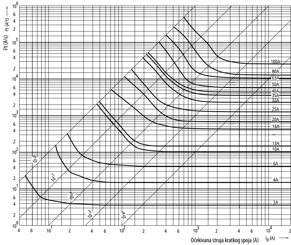
Diagram I t t karakteristika
