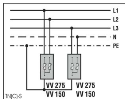
Slika 11: Primer vezave TNS sistema
