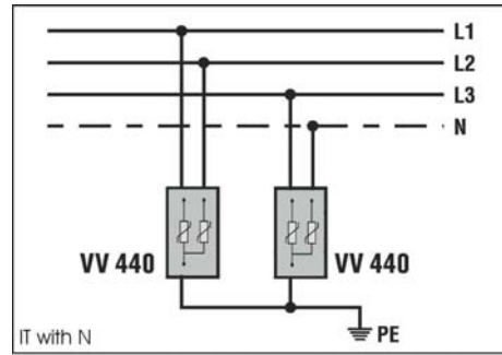
Slika 13: Primer vezave IT sistema
