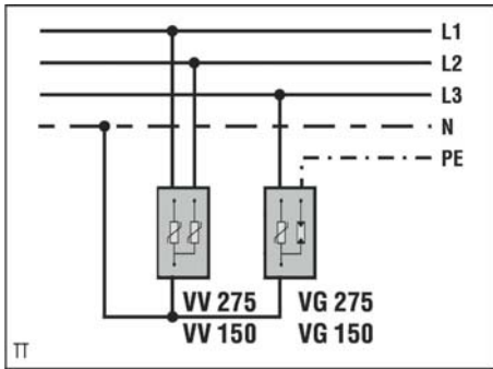
Slika 12: Primer vezave TT sistema
