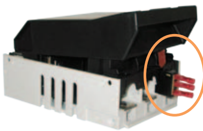
MST 00 1p+3p mikro stikalo za indikacijo odprtja ločilnika
